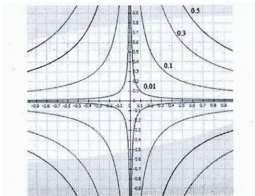
Рис. 3. Линии уровня мультипликативной ОФ.
