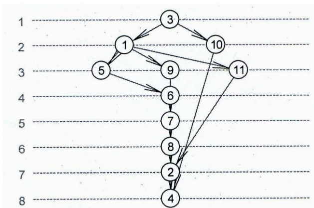
Рис. 5. Граф доминирования для рассмотренного примера.
