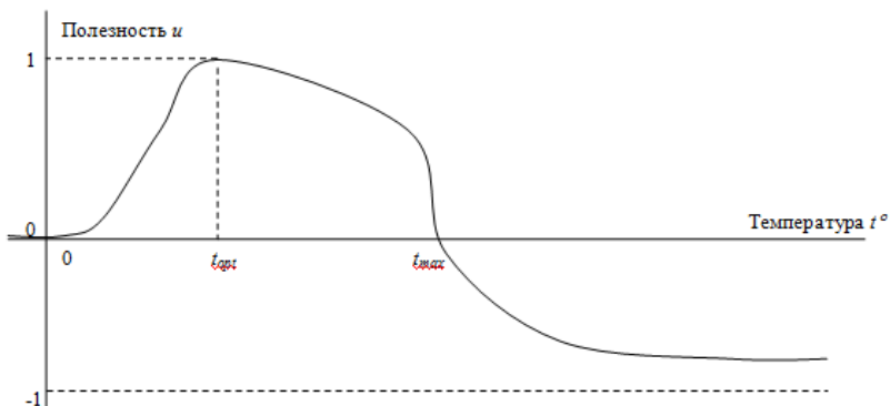
Рис. 1. Пример знакопеременной функции полезности.
