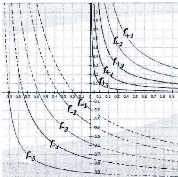
Рис. 4. Примерный ожидаемый вид линий уровня.
