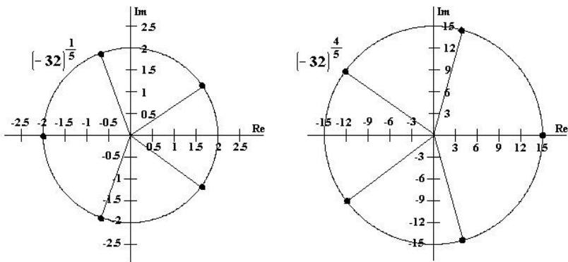
Рис. 2. Корни отрицательных чисел.
