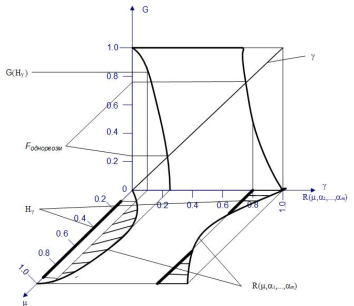
Рис. 3. Графическая интерпретация нахождения показателя возможности безотказной работы немонотонных однородных структур
