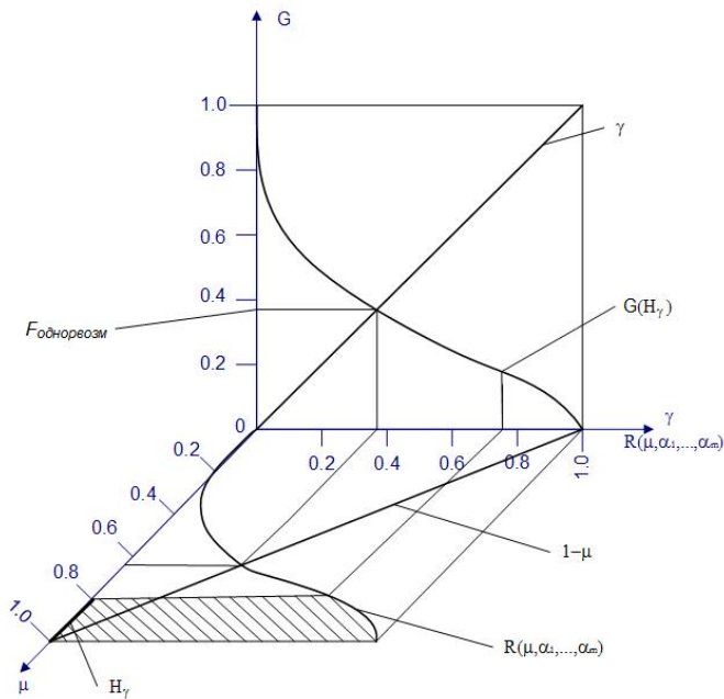
Рис. 2. Графическая интерпретация нахождения показателя возможности безотказной работы однородных структур
