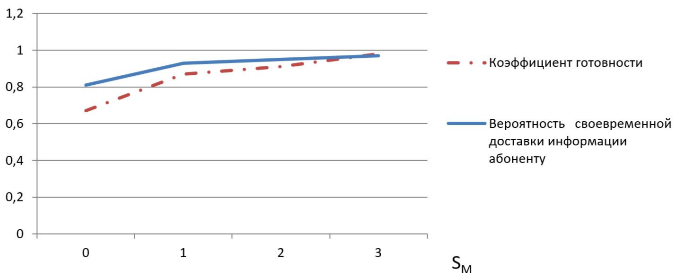
Рис. 2. Графики показателей качества ССПД в зависимости от глубины мониторинга
